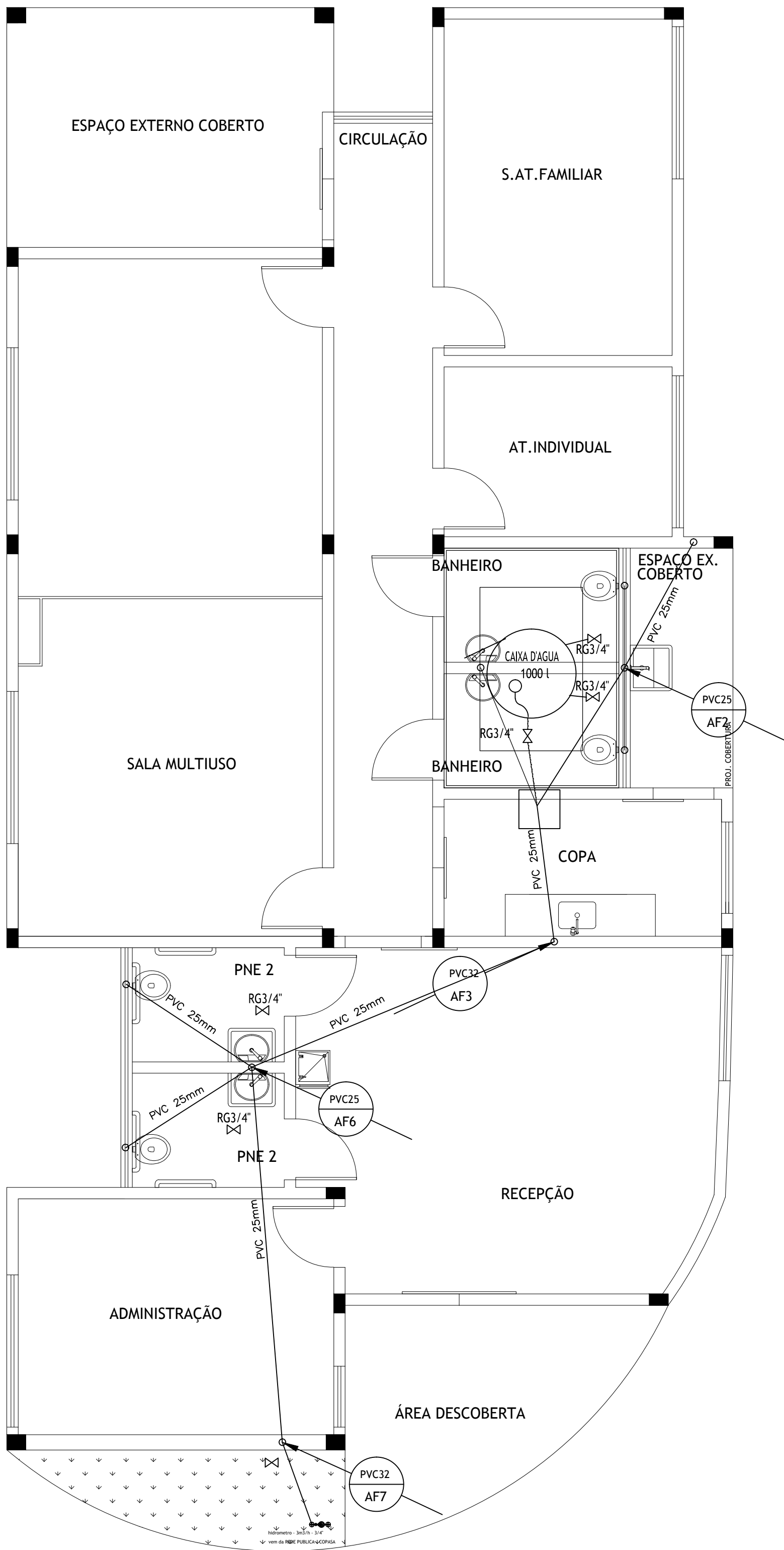
PL. PAVTO TÉRREO - HIDRÁULICA ESCALA= 1: 50
