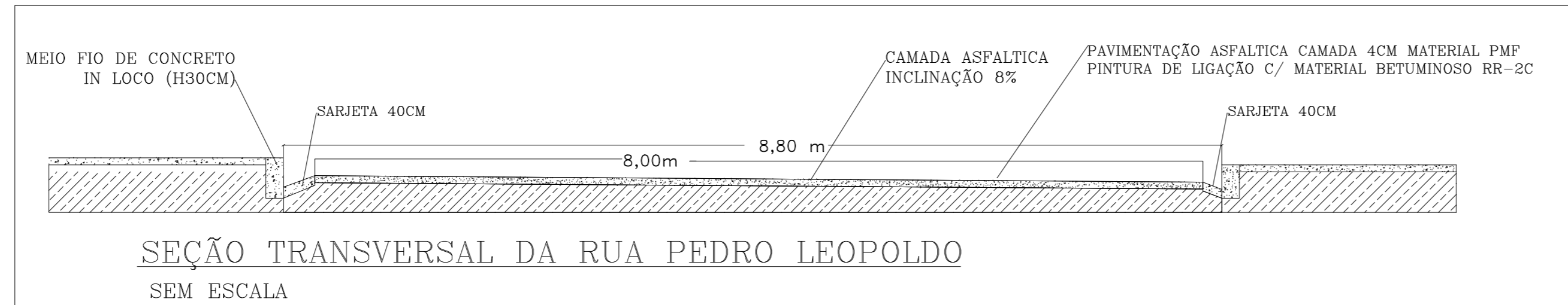
CORTE ESQUEMÁTICO
