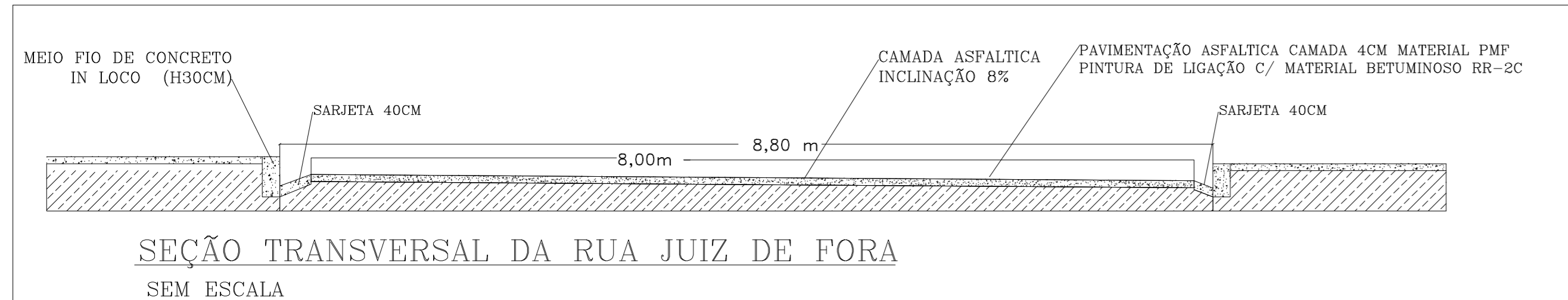
CORTE ESQUEMÁTICO
